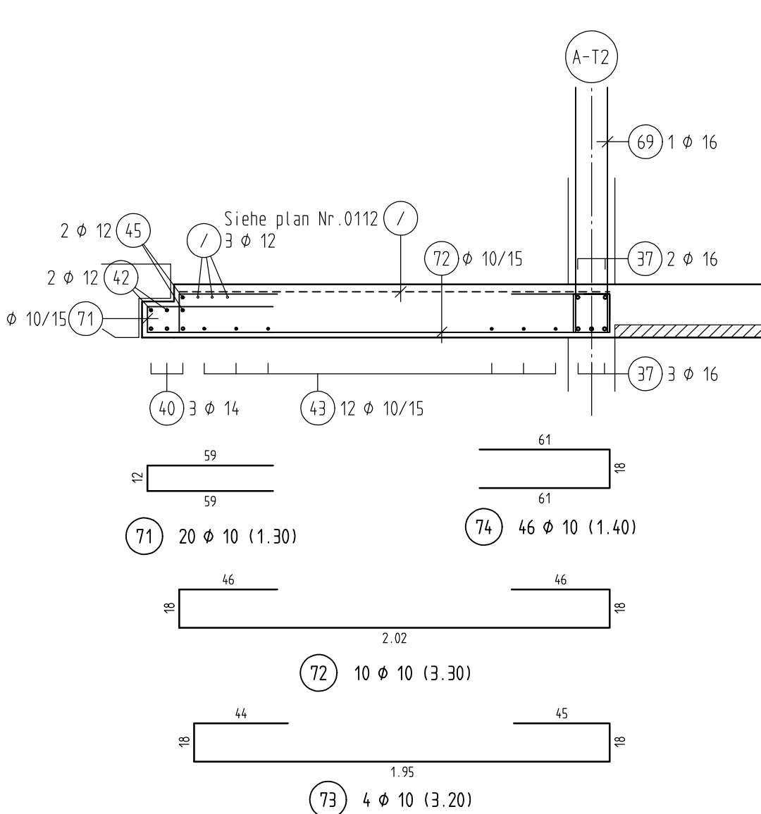
SNITT 11-11, M=1:25
