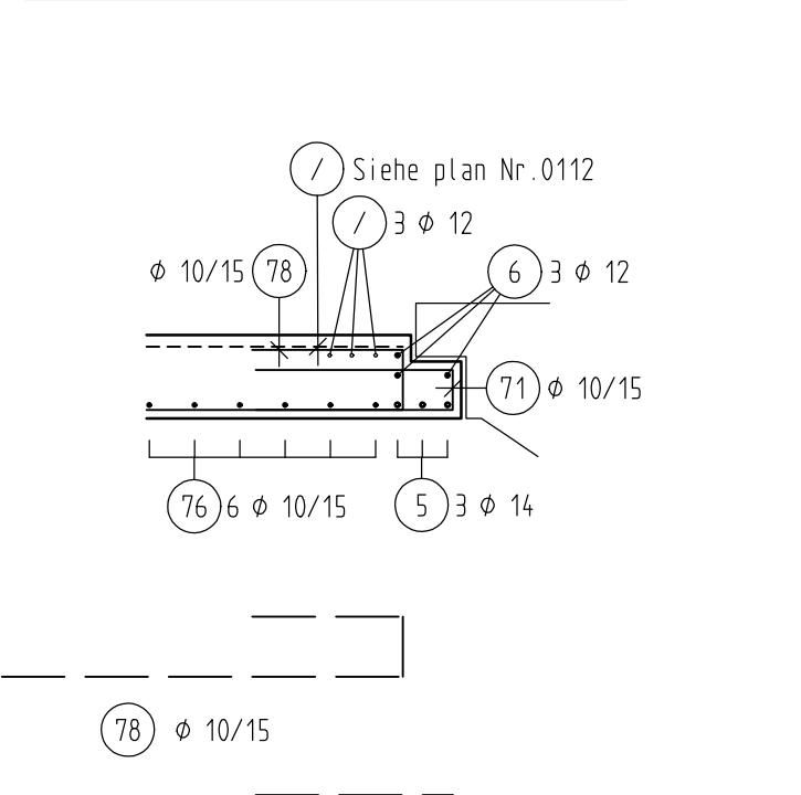
SNITT 10-10, M=1:25
