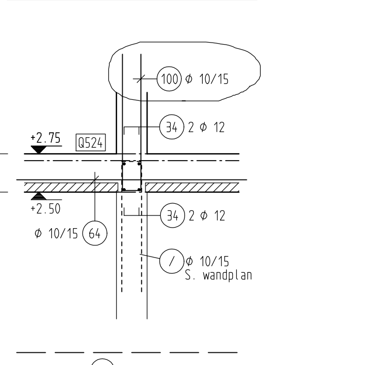
SNITT 7-7, M=1:25
