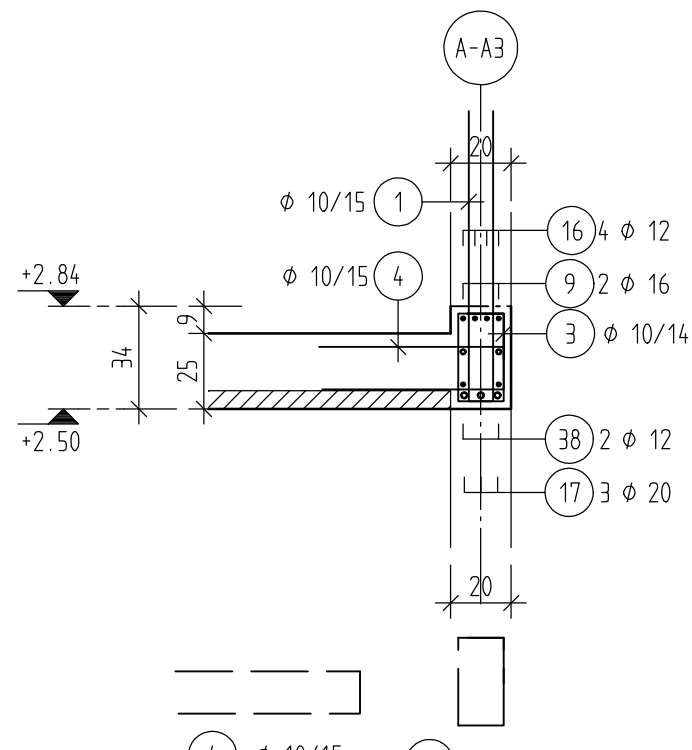
SNITT 3-3, M=1:25
