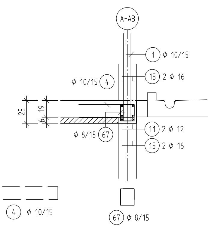
SNITT 2-2, M=1:25
