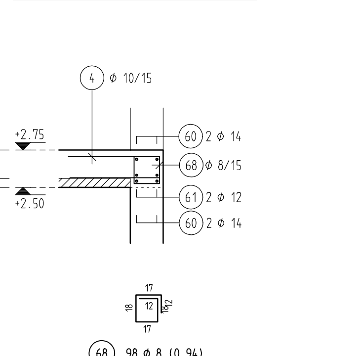
SNITT 9-9, M=1:25
