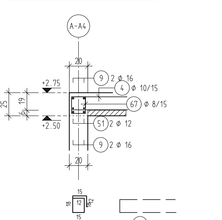
SNITT 6-6, M=1:25
