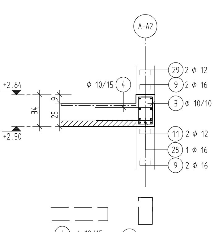
SNITT 4-4, M=1:25
