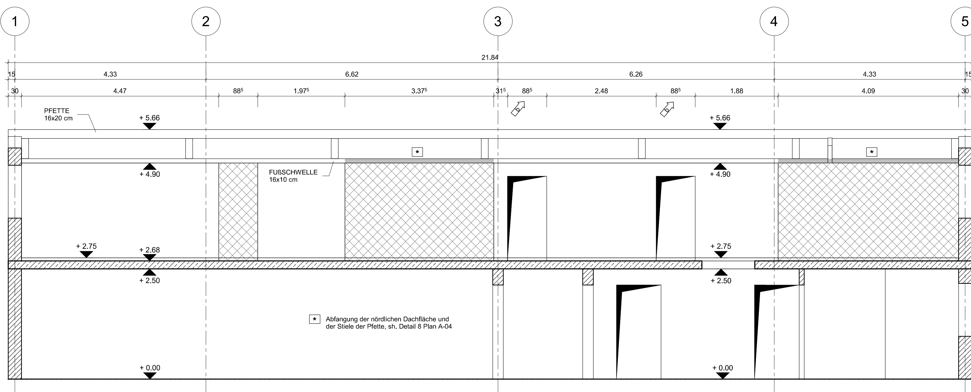
SNITT A-A, M.=1:50
