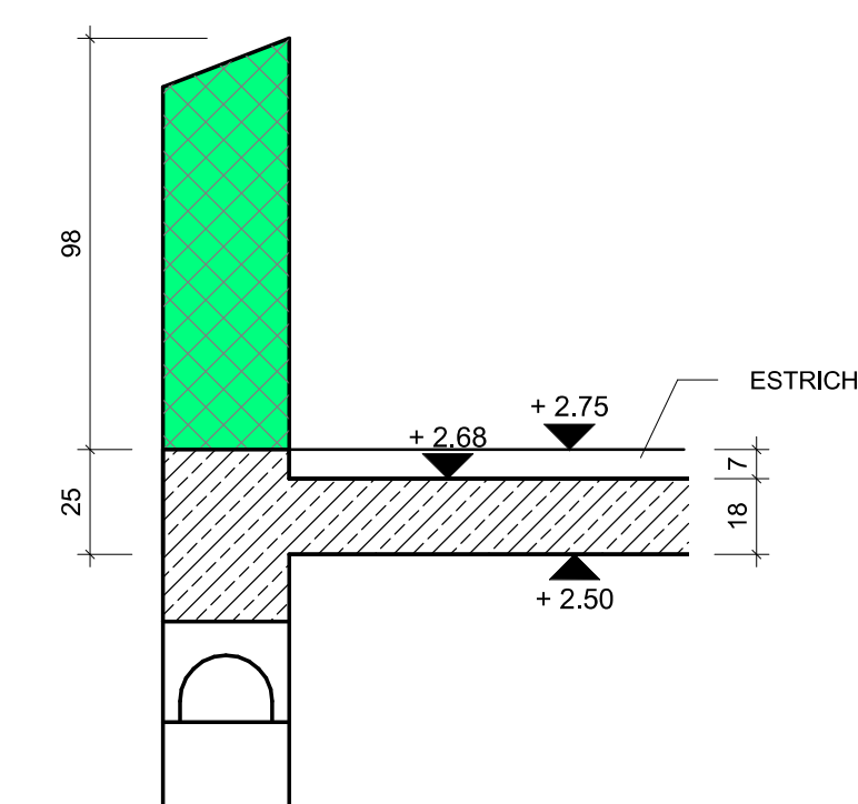
SNITT B-B, M.=1:20
