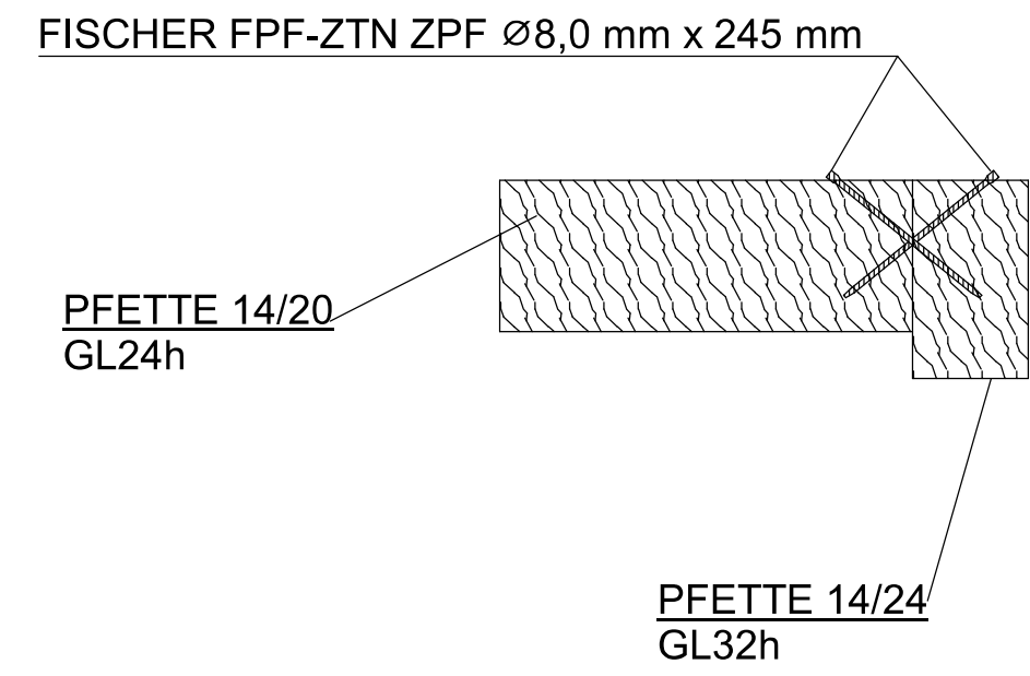
ANSCHLUSS A2 M.=1:10
