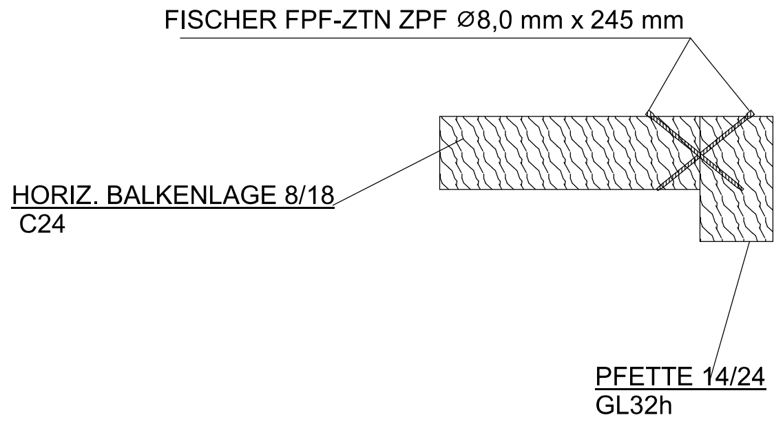
ANSCHLUSS A2 M.=1:10
