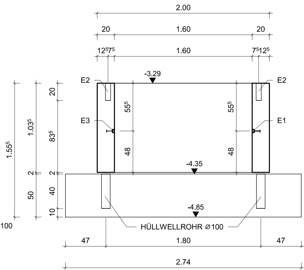
W2 , M=1:25
