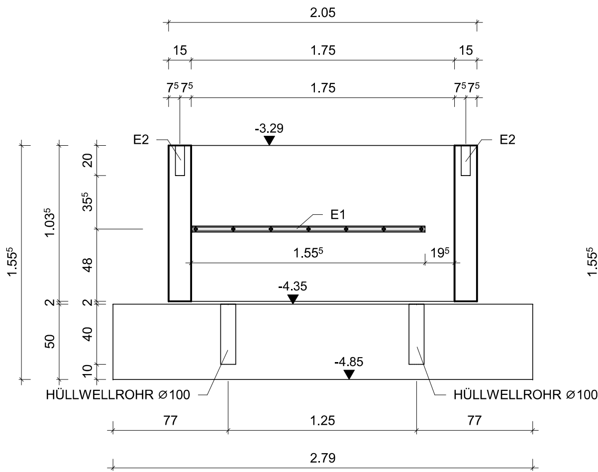
W1 , M=1:25
