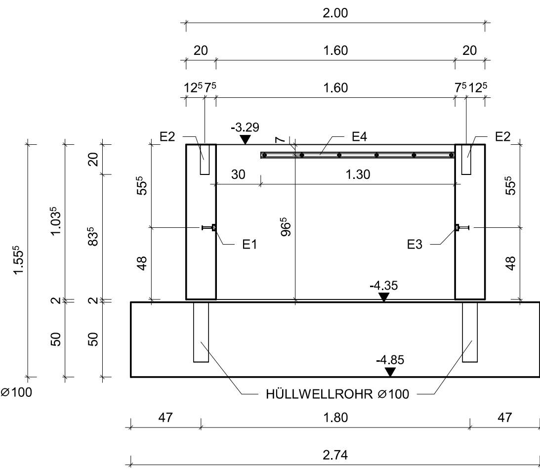
W4 , M=1:25
