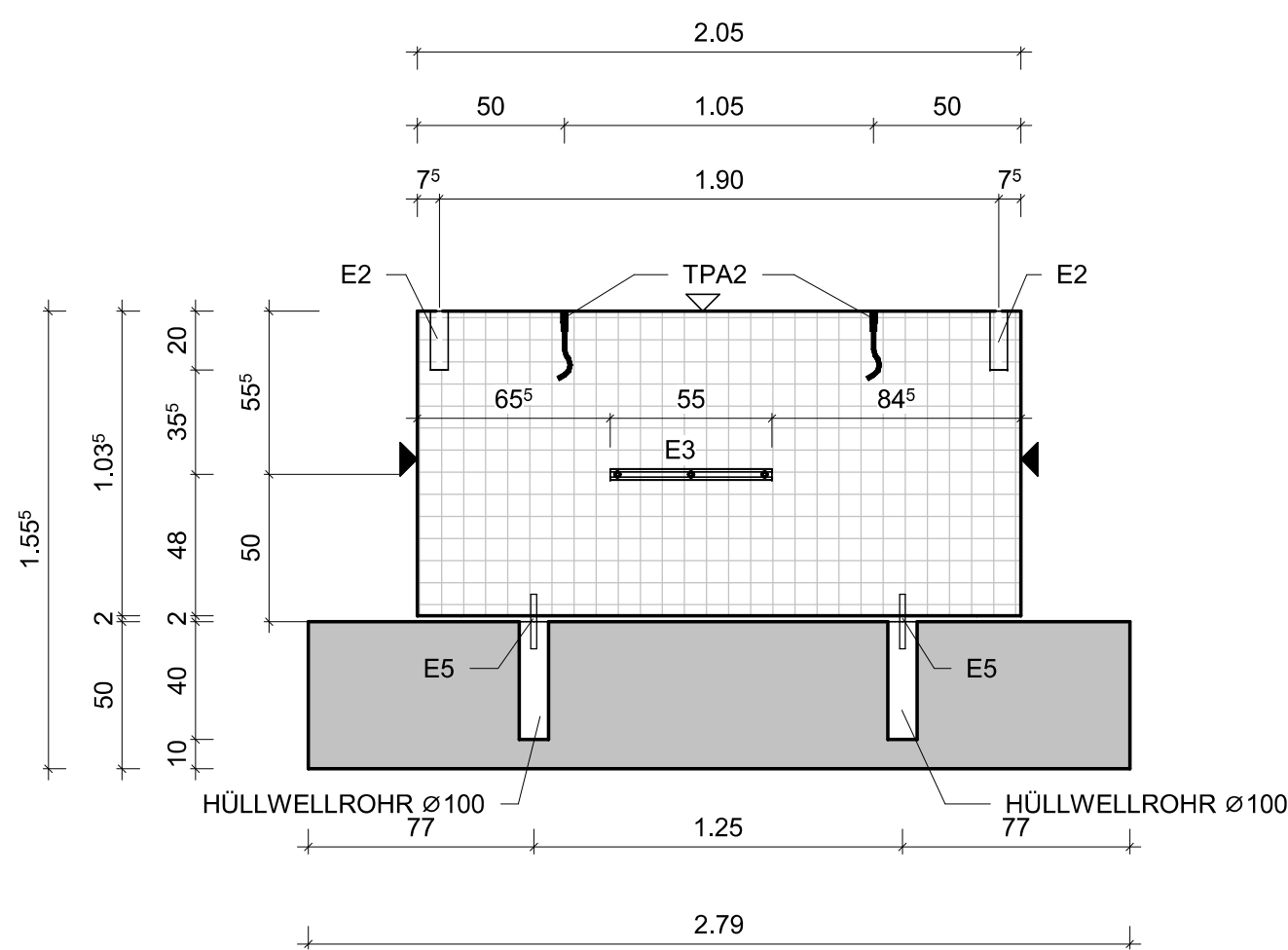
SCHNITT 1-1 , M=1:25
