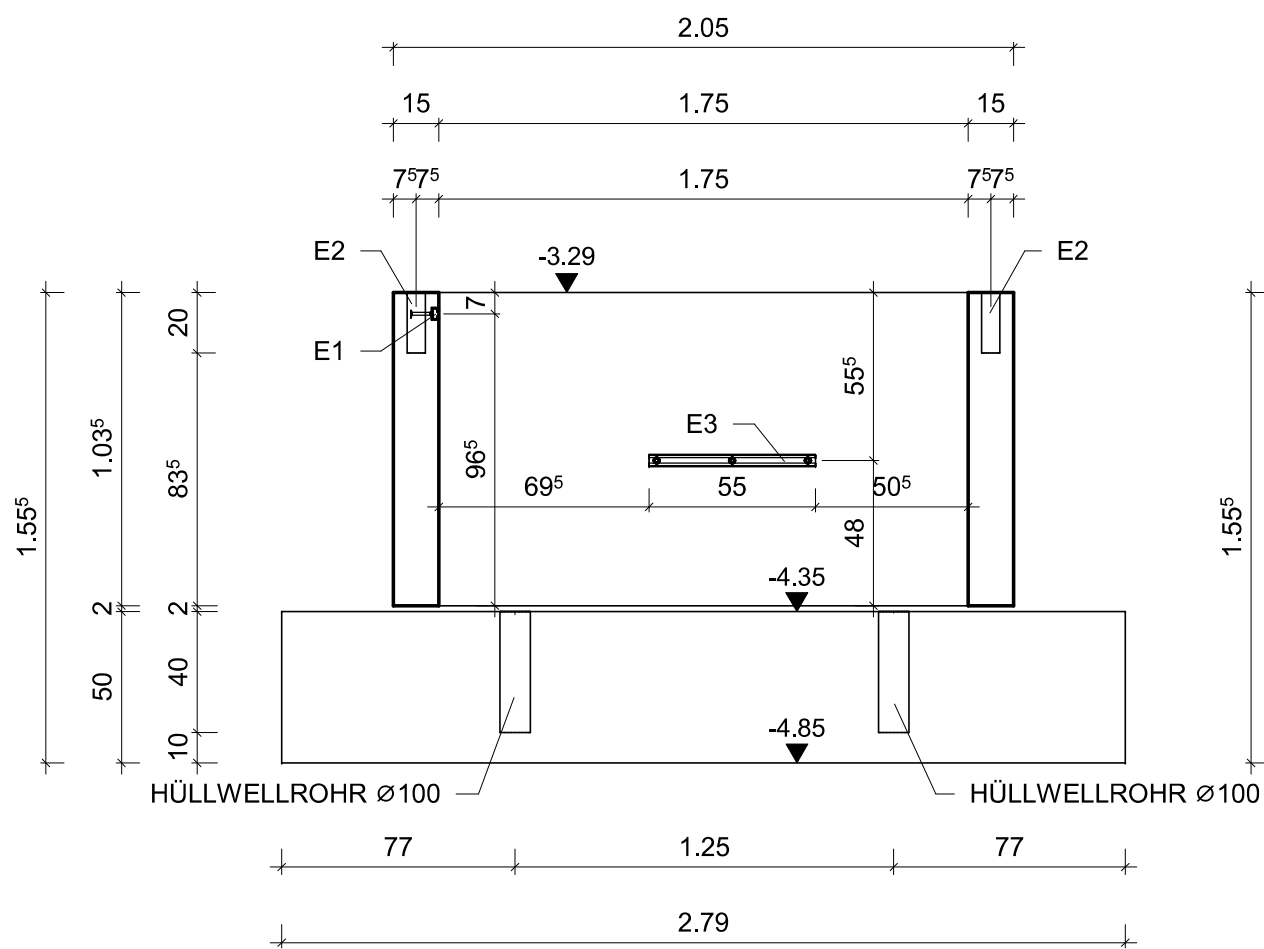
W3 , M=1:25
