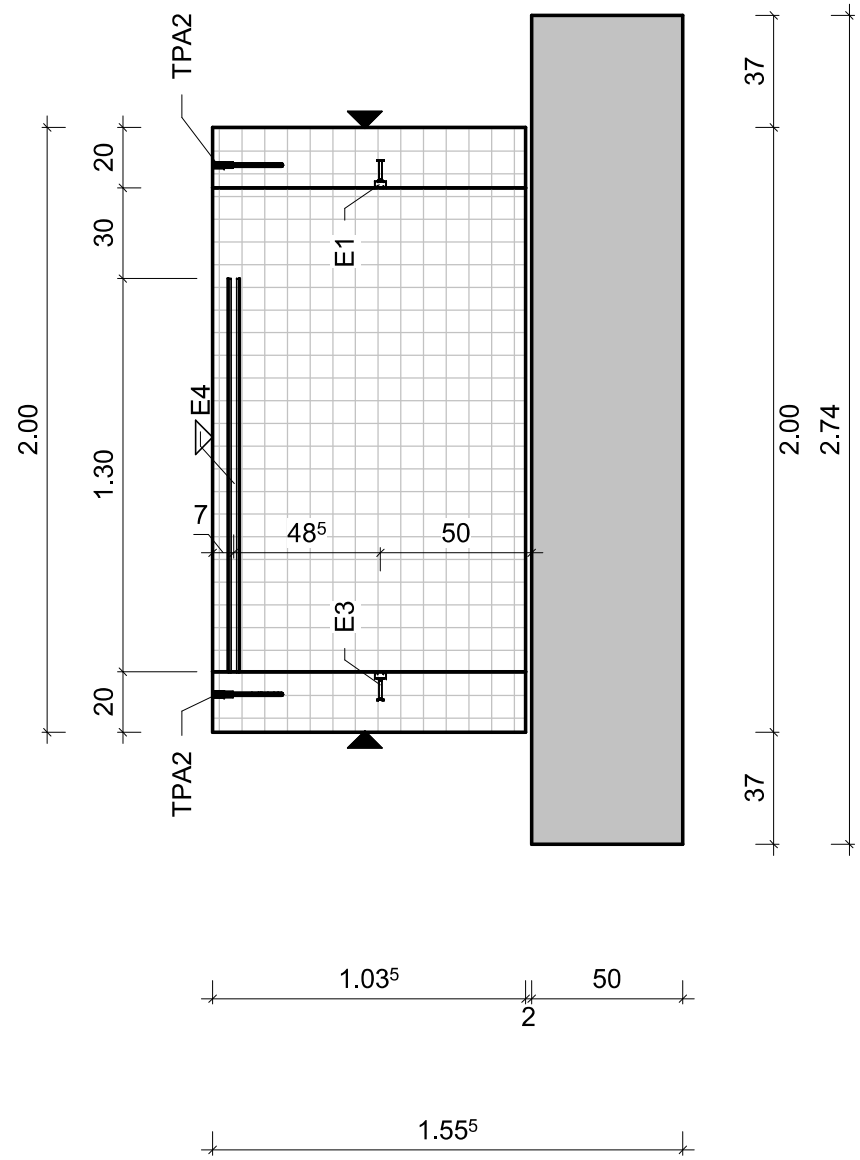
SCHNITT 2-2 , M=1:25
