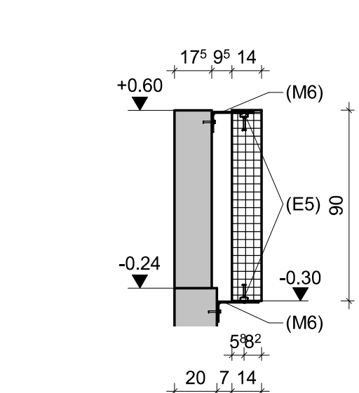
SCHNITT 4-4 , M=1:25
