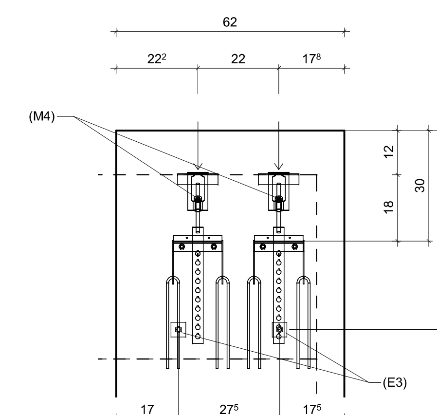
DETAIL "B" 1x UND 1x GESPIEGELT, M=1:10
