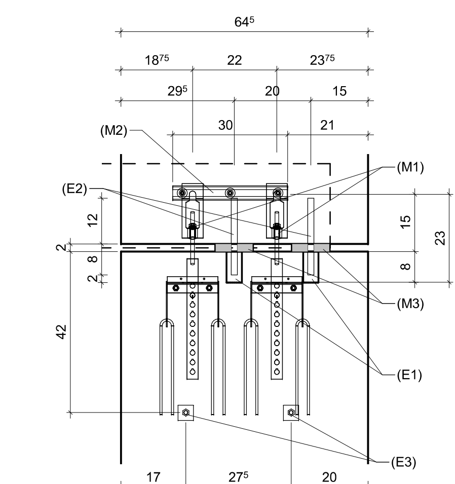
DETAIL "A" 3x UND 3x GESPIEGELT , M=1:10
